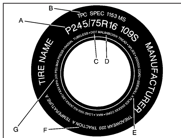
Exemple d'un pneu de tourisme (grandeur « P-Metric »)
