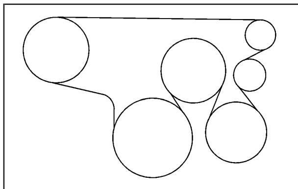
Moteur L5 de 3,7 L
