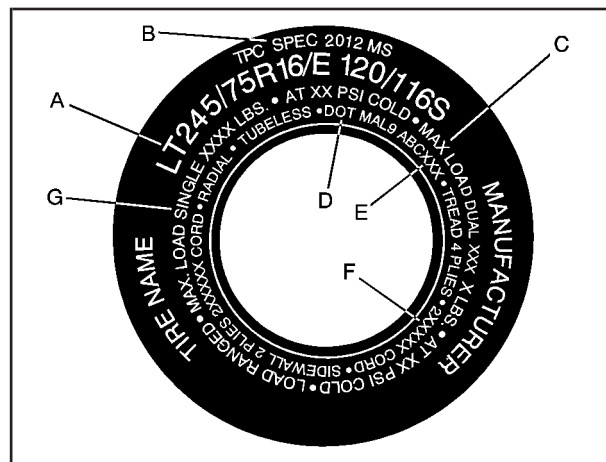
Exemple d'un pneu de camionnette (grandeur « LT-Metric »)
