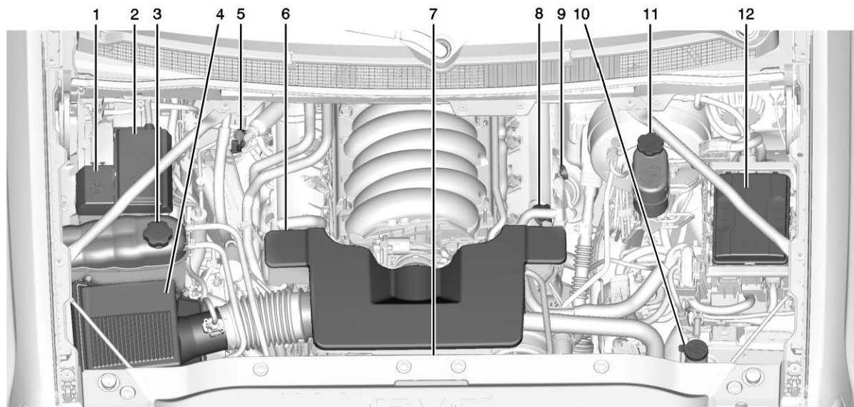
Moteur 5.3L de Tahoe/Suburban 6 vitesses
