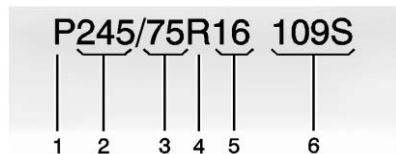
Pneu de tourisme (grandeur « P-Metric »)
