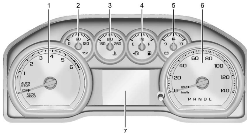
Groupe d'instruments de base - unité anglaise illustrée, unités métriques similaires
