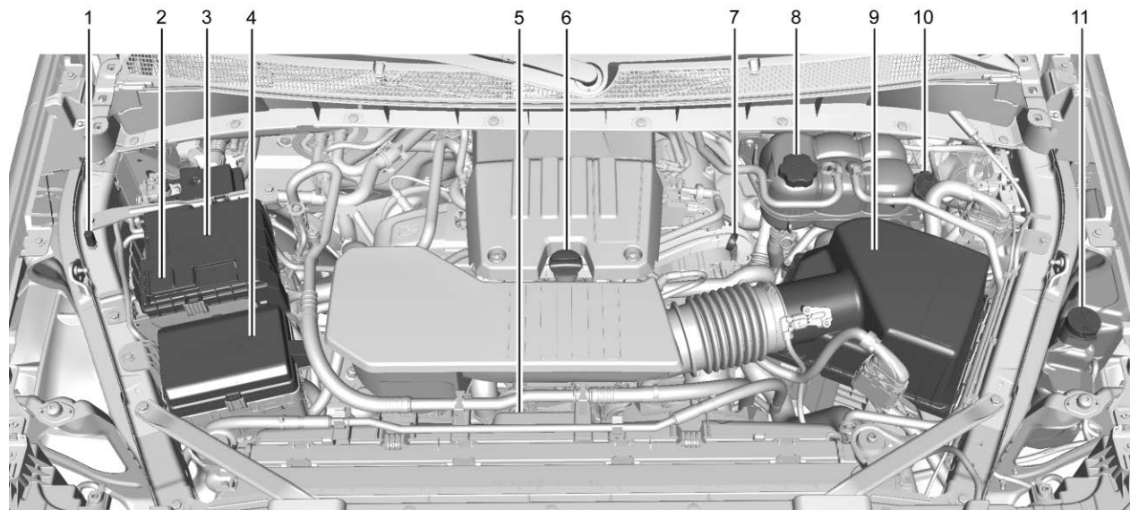
Moteur 2.7L I4 (L3B)
